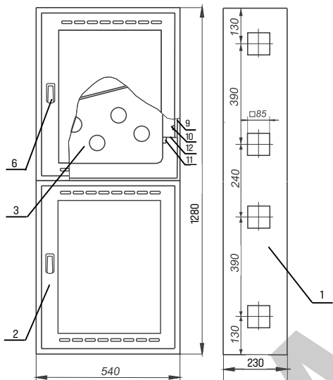
Рисунок 1 - Шкаф пожарный ПРЕСТИЖ-03-Н
