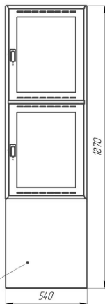
Рисунок 3 - Шкаф пожарный «ПРЕСТИЖ» приставной
