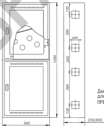
Рисунок 1- Шкафы пожарные «ПРЕСТИЖ» навесные
